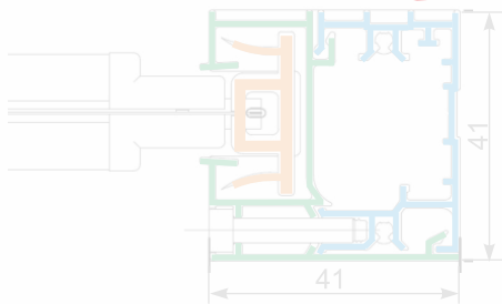
Przekrój prowadnicy
