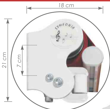
Montaż ścienny
