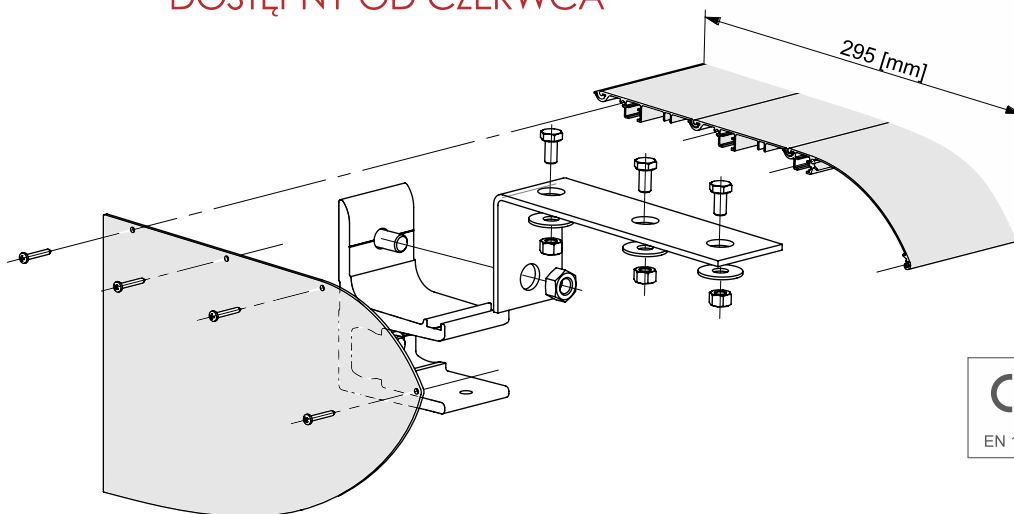
Daszek przed złożeniem PAKIET
